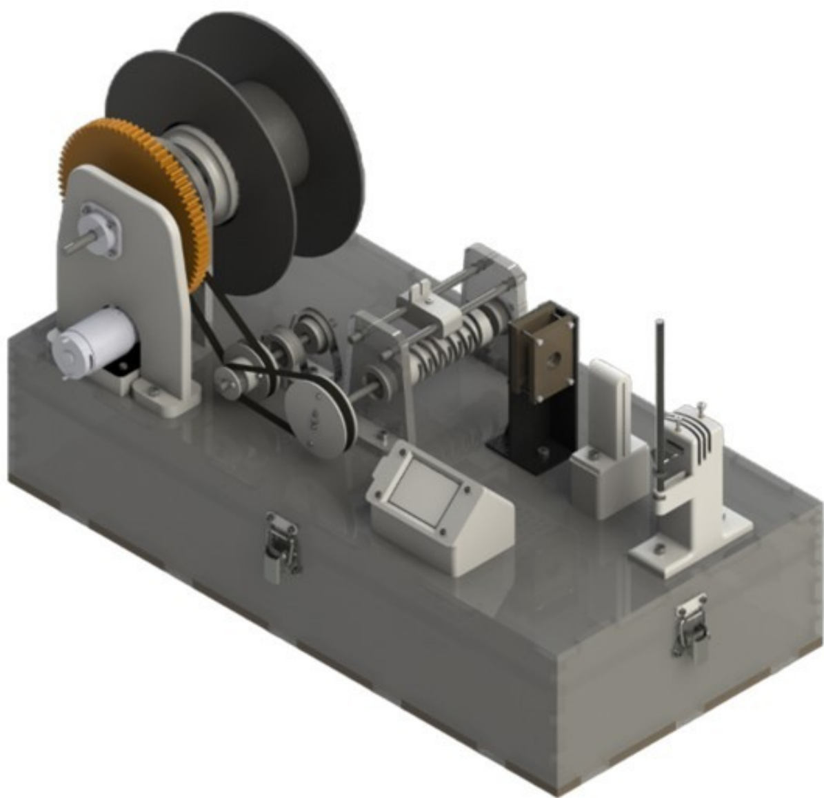
Gambar 1 - Tampak Perspektif
